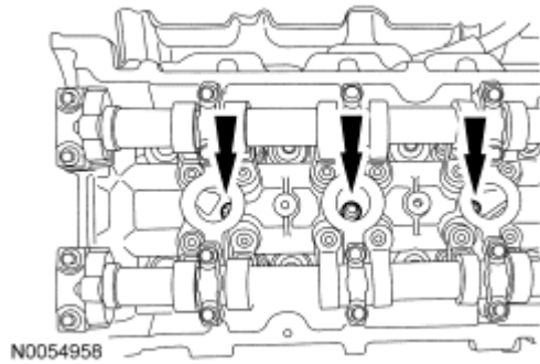
Fig. 294: Spark Plugs
