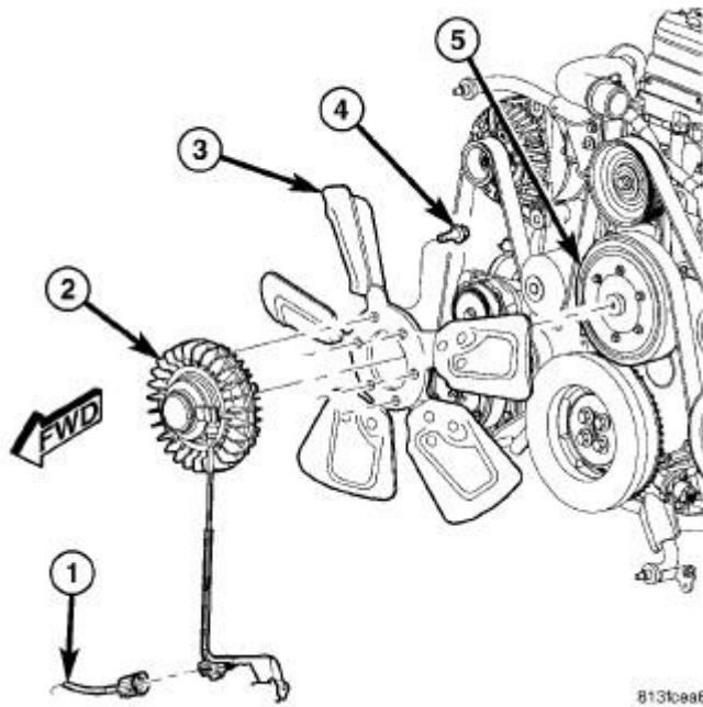
Fig. 338: Fan Blade/Viscous Fan Drive Courtesy of CHRYSLER LLC
