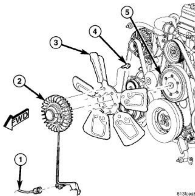
Fig. 344: Fan Blade/Viscous Fan Drive Courtesy of CHRYSLER LLC
