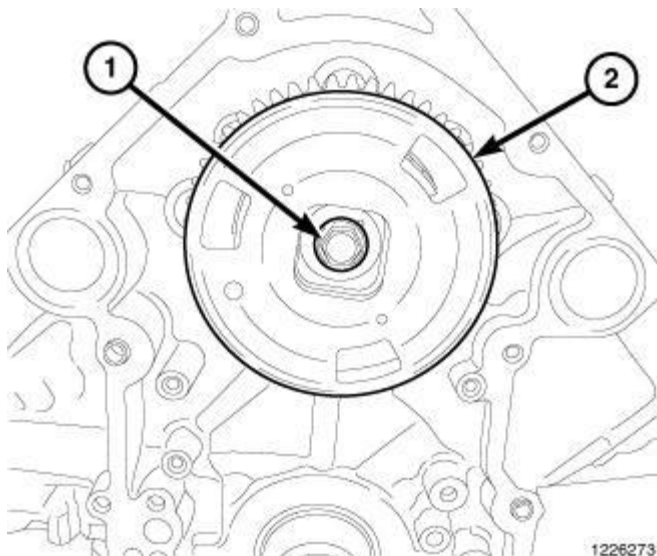
Fig. 125: Camshaft Phaser & Bolt
