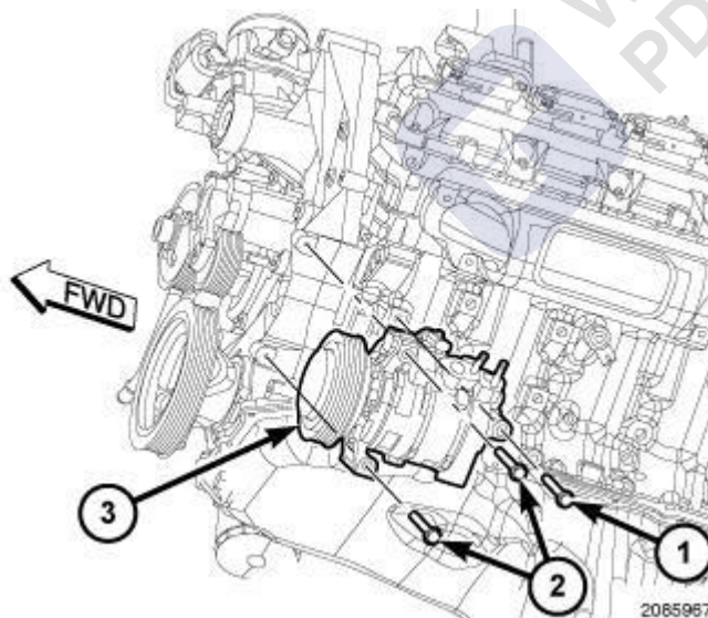
Fig. 384: A/C Compressor
