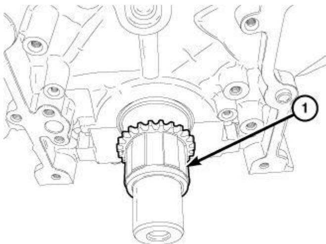
Fig. 341: Crankshaft Sprocket
