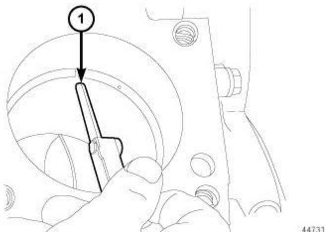
Fig. 195: Piston Ring End Gap
