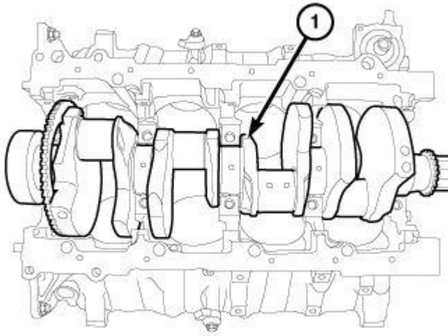
Fig. 169: Crankshaft
