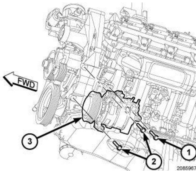
Fig. 384: A/C Compressor
