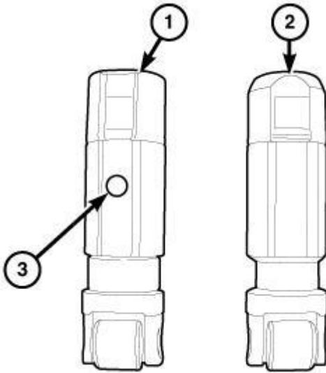
Fig. 50: MDS Lifter
