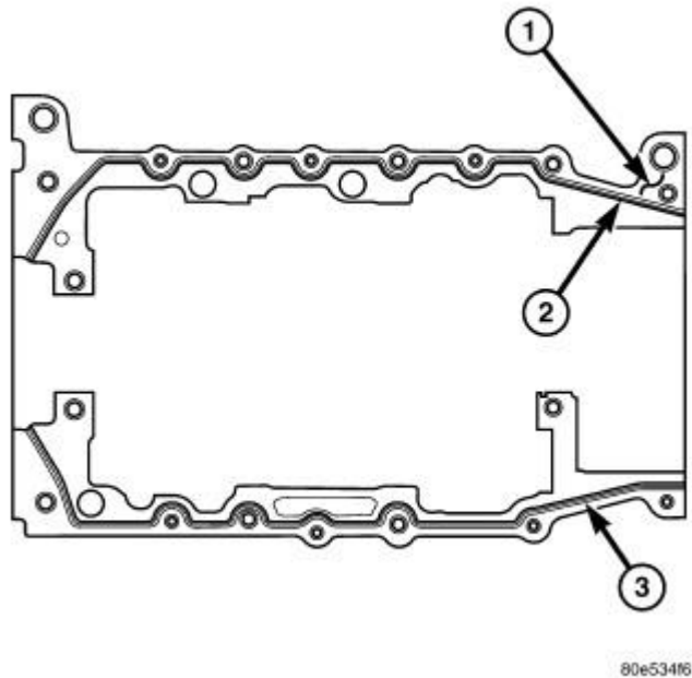
Fig. 81: Bedplate Sealant
