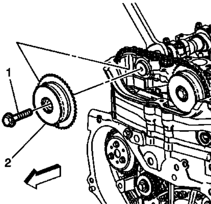
Fig. 91: Camshaft Actuator
