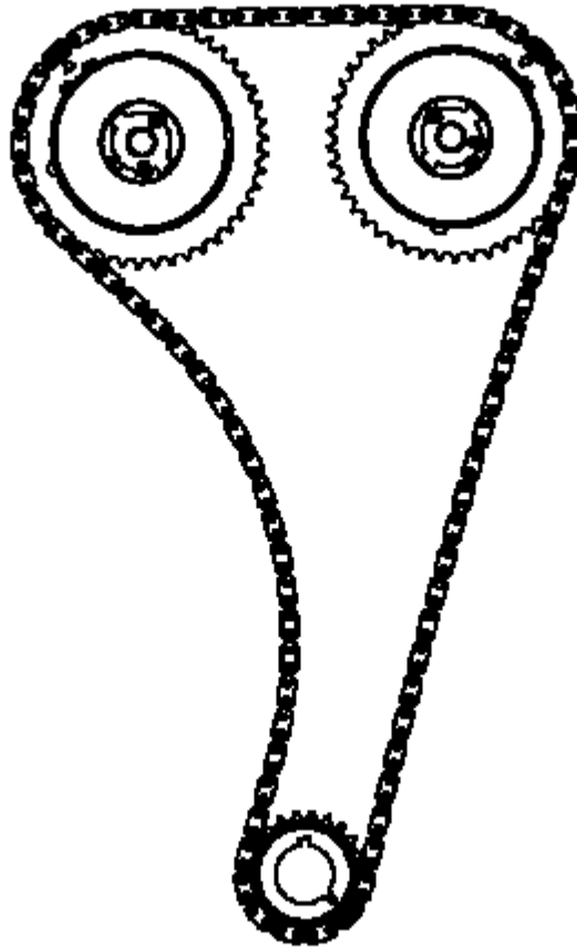
Fig. 81: Chain And Sprockets
