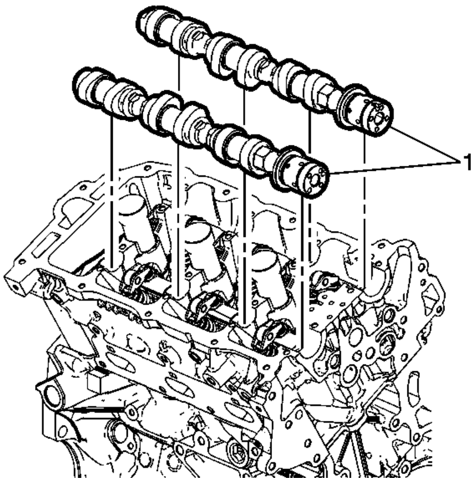
Fig. 137: Camshafts
