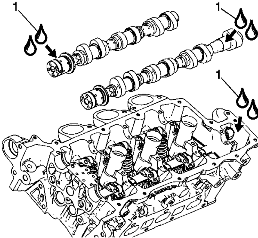
Fig. 128: Camshaft Journal Lubrication Points
