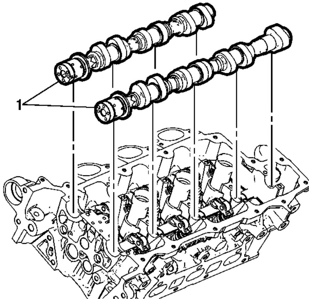
Fig. 126: Camshafts
