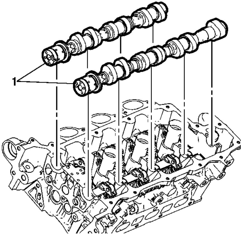
Fig. 126: Camshafts
