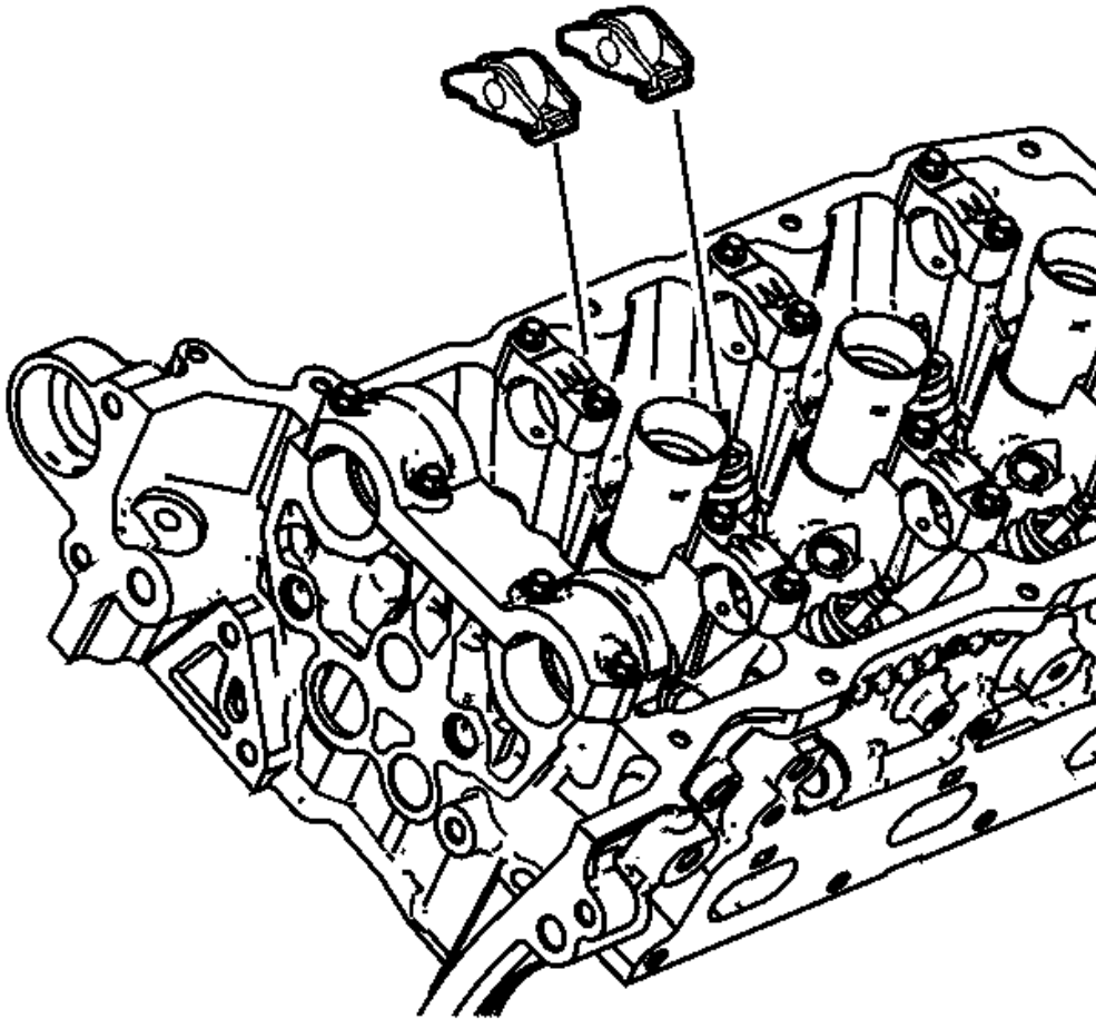
Fig. 148: Valve Rocker Arms
