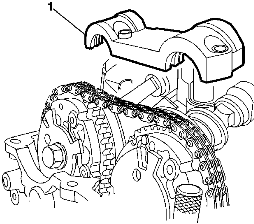
Fig. 89: Camshaft Front Cap
