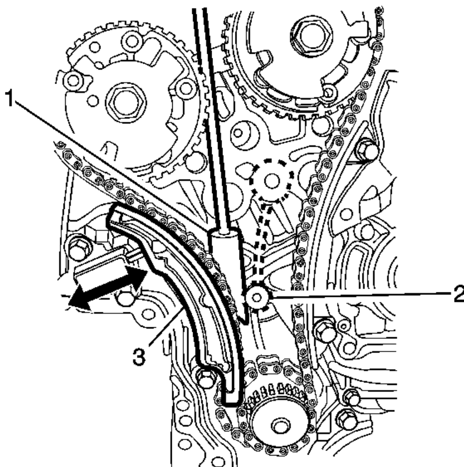
Fig. 110: Retainer Wedge
