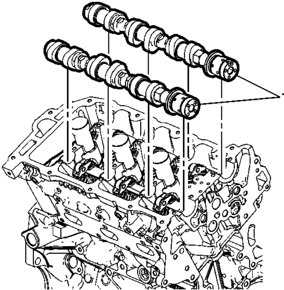
Fig. 168: Camshafts
