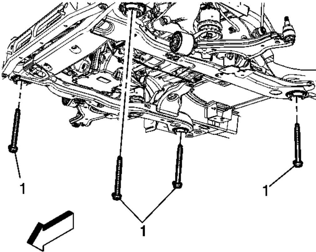
Fig. 265: Frame-To-Body Bolts
