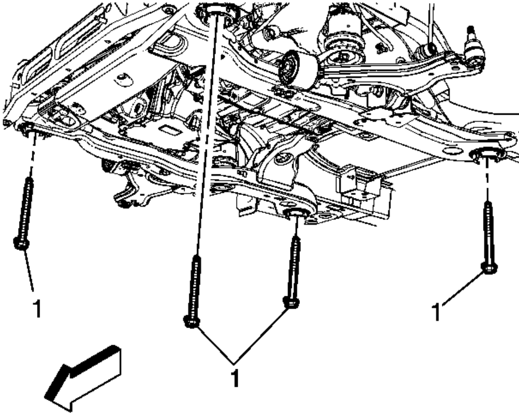
Fig. 241: Frame-To-Body Bolts
