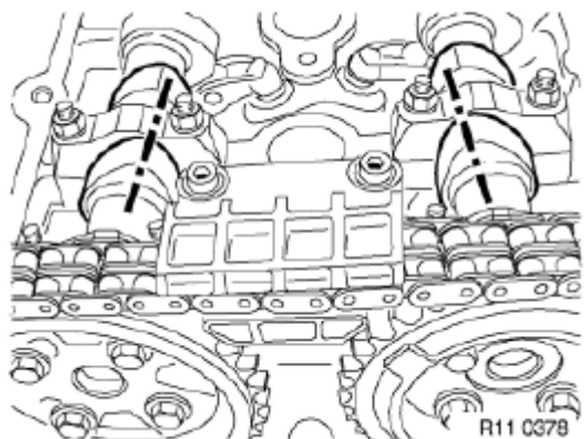
Fig. 216: Aligning Camshafts
