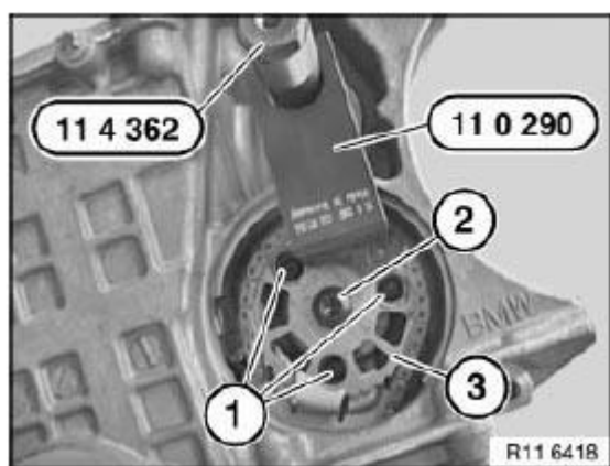
Fig. 377: Turning Sprocket
