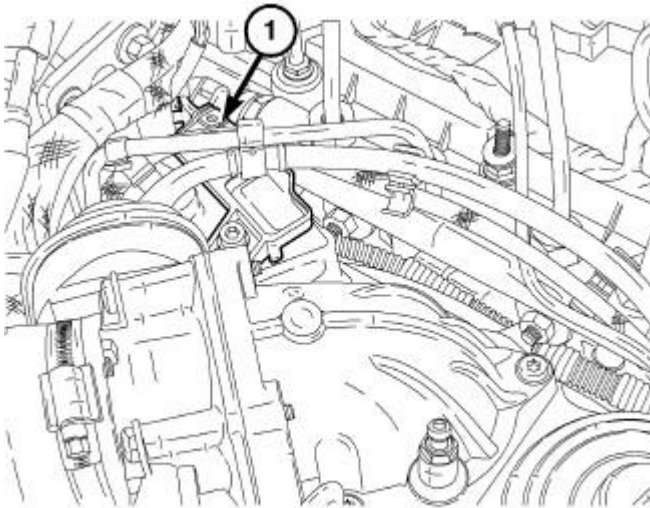
Fig. 19: IAT/BPS SENSOR
