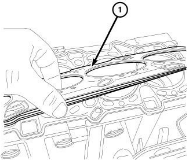
Fig. 57: MLS GASKET
