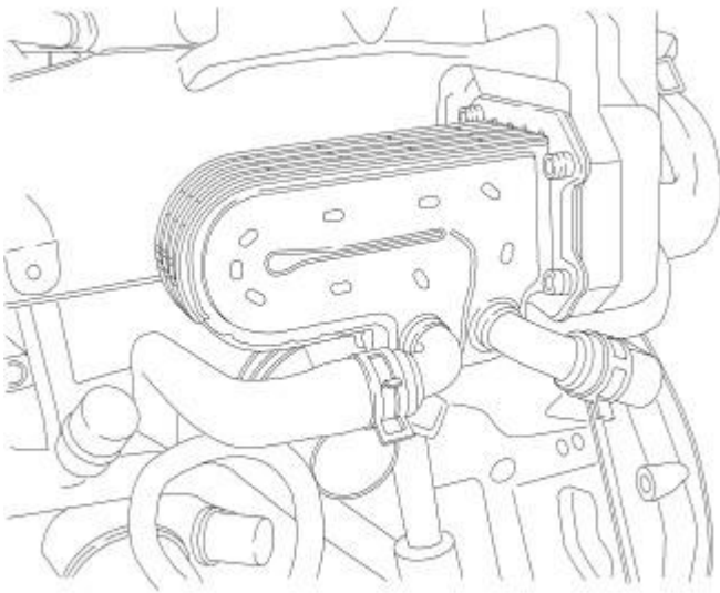
Fig. 273: EGR COOLER
