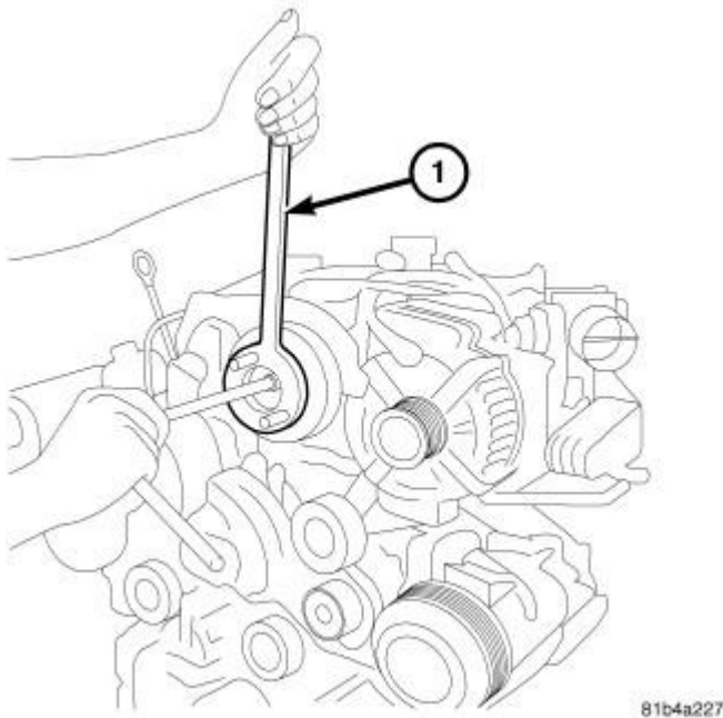
Fig. 358: REMOVE CAMSHAFT SPROCKET BOLT
