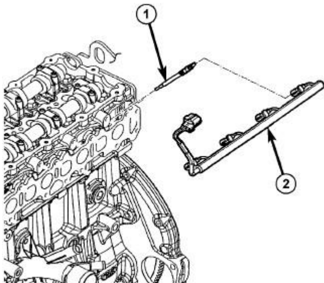
Fig. 290: Glow Plugs & Wiring Harness
