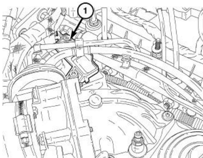
Fig. 283: IAT/BPS SENSOR
