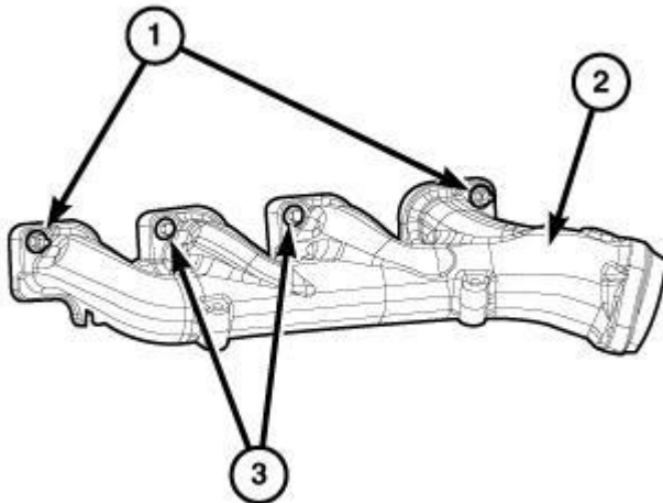
Fig. 388: Exhaust Manifold, Stud & Bolts
