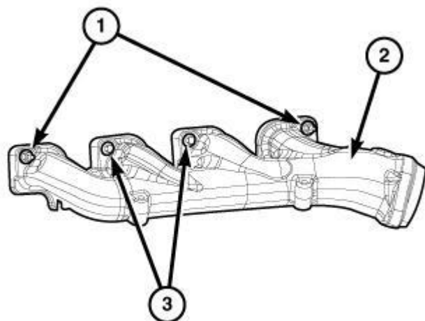
Fig. 391: Exhaust Manifold, Stud & Bolts
