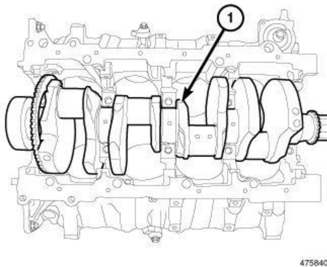
Fig. 194: Crankshaft
