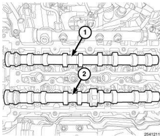
Fig. 127: Camshafts
