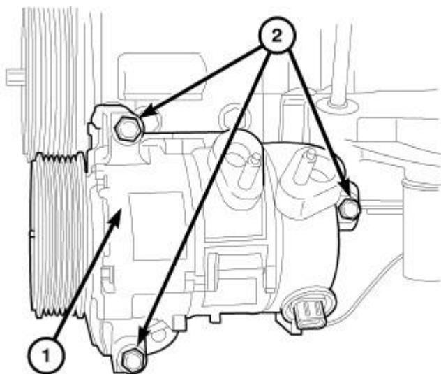
Fig. 329: A/C Compressor - R & I
