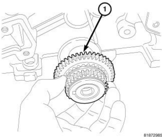
Fig. 381: Crankshaft Sprocket
