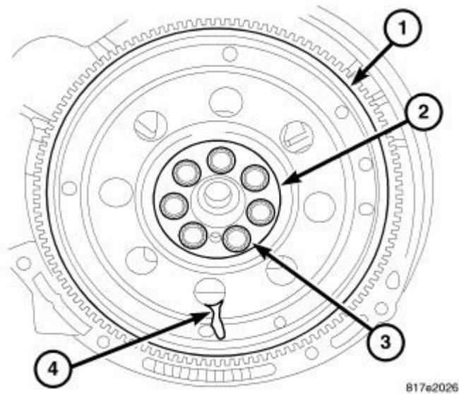
Fig. 271: Flex Plate
