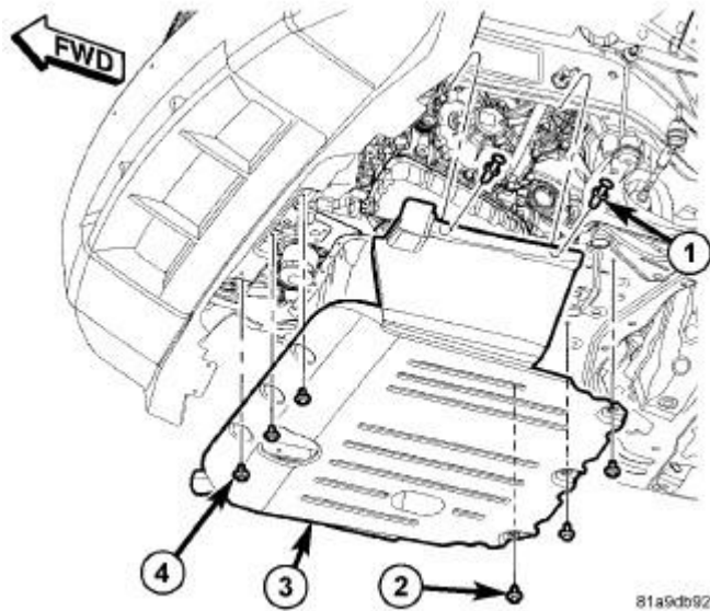
Fig. 315: Belly Pan
