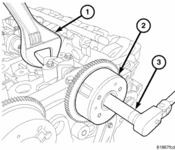
Fig. 173: CAMSHAFT PHASER
