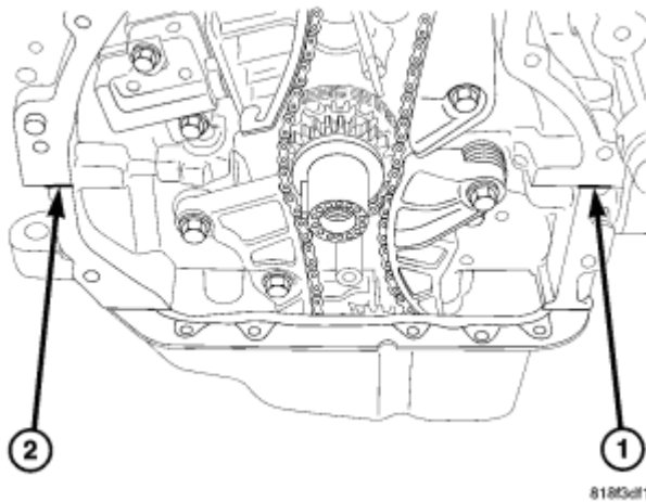
Fig. 387: Lower T-Joints
