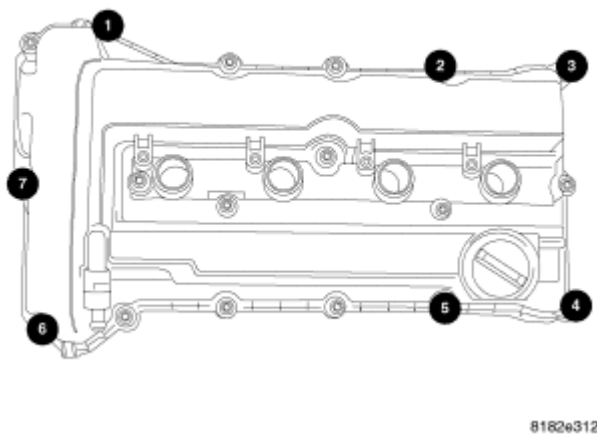
Fig. 155: Stud Location
