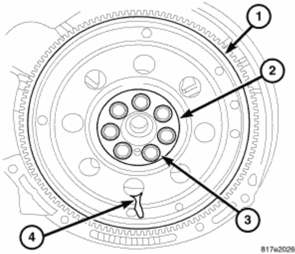
Fig. 195: Flex Plate
