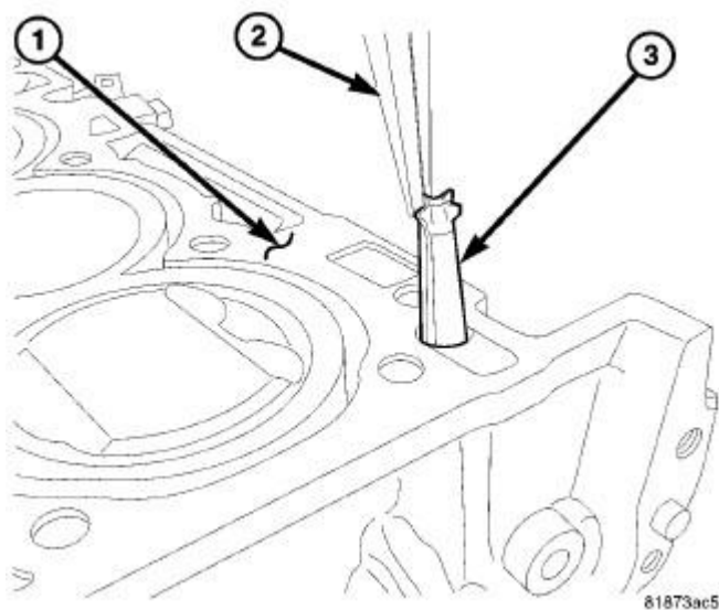
Fig. 106: VVT Filter
