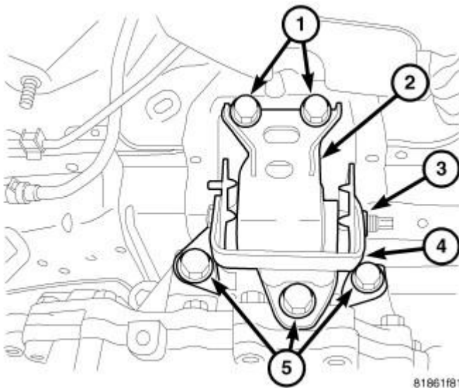
Fig. 194: LEFT MOUNT
