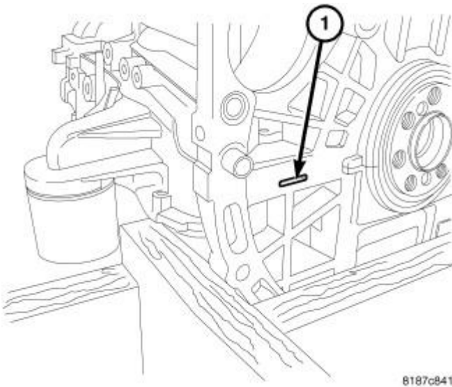
Fig. 241: PRY POINT 1
