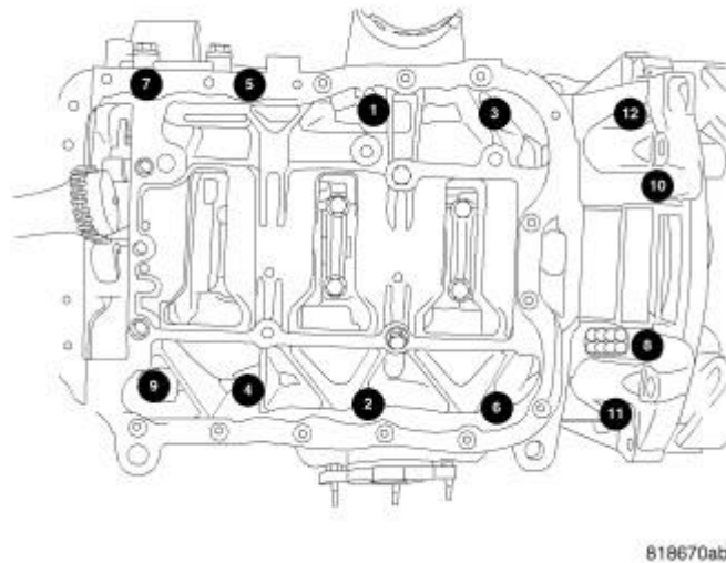
Fig. 244: LADDER FRAME TORQUE
