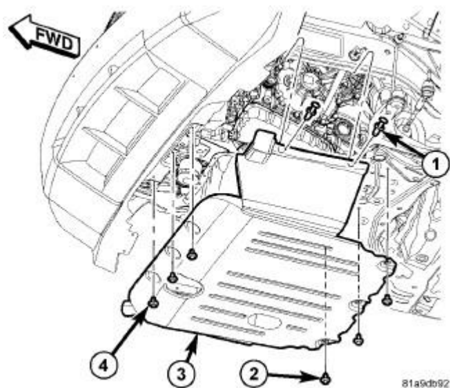
Fig. 369: Belly Pan
