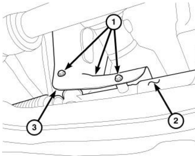
Fig. 367: Gear Shield
