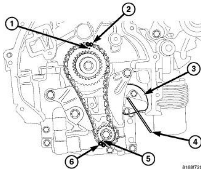
Fig. 319: BSM TENSIONER
