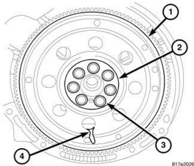
Fig. 239: FLEX PLATE
