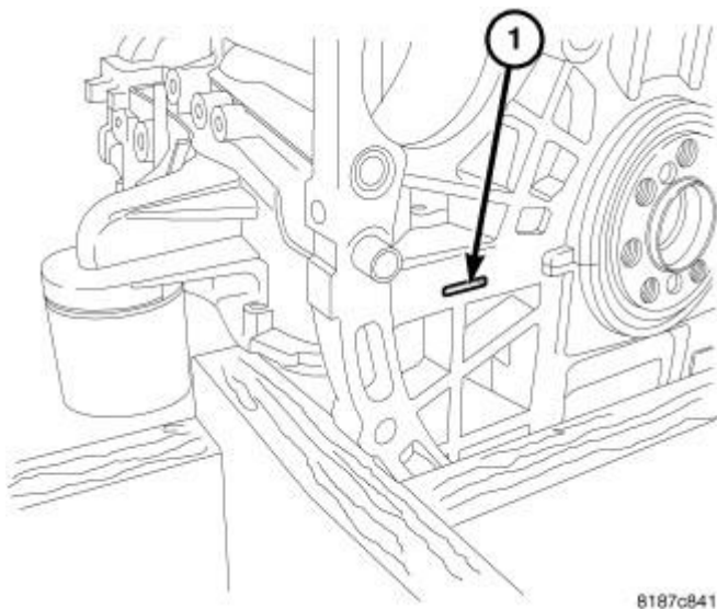
Fig. 216: Pry Point 1
