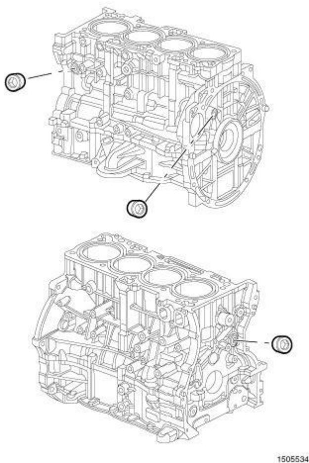
Fig. 299: Tapered Plugs
