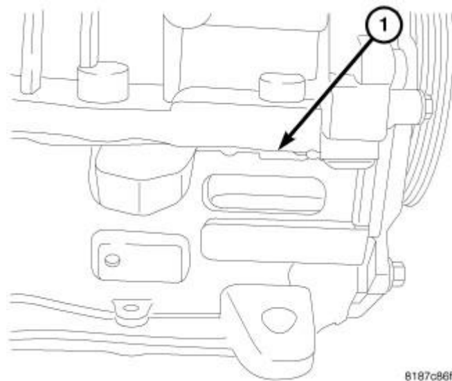
Fig. 217: Pry Point 2
