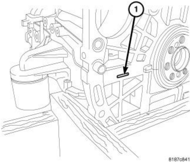
Fig. 219: PRY POINT 1
