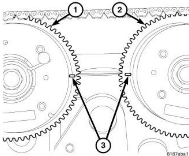
Fig. 346: Camshaft Timing
