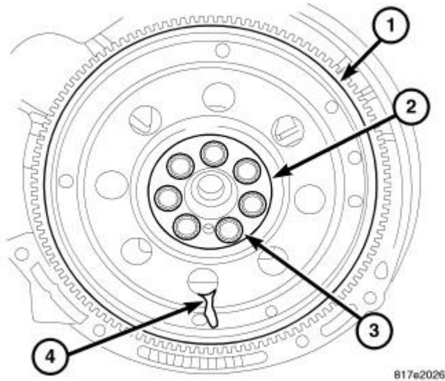
Fig. 241: FLEX PLATE
