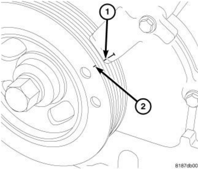
Fig. 345: TDC
