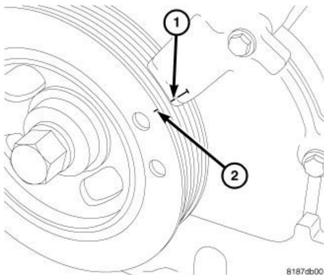
Fig. 347: TDC
