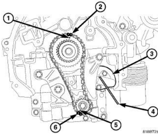
Fig. 306: BSM Tensioner
