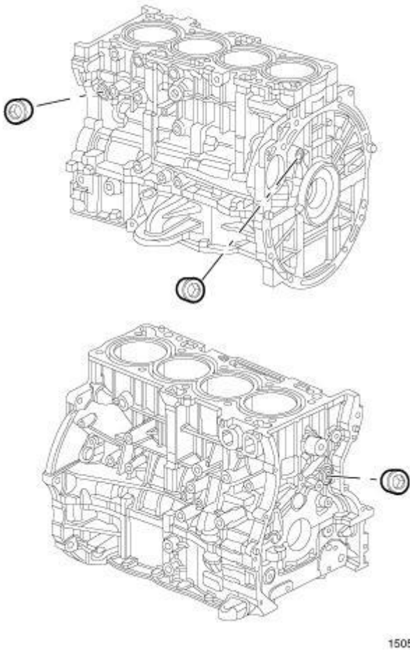
Fig. 301: Tapered Plugs
