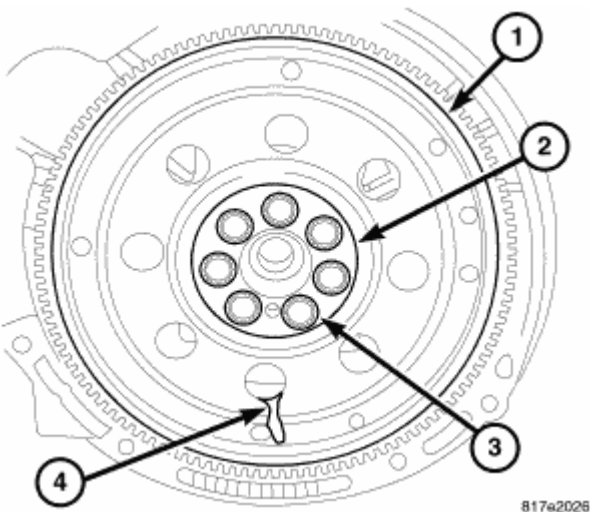
Fig. 173: Flex Plate
