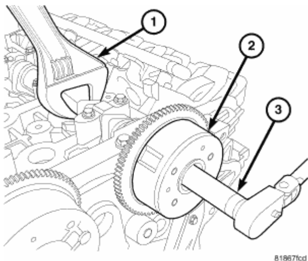
Fig. 167: CAMSHAFT PHASER
