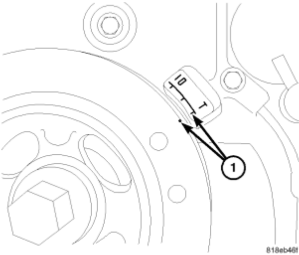
Fig. 159: TDC
