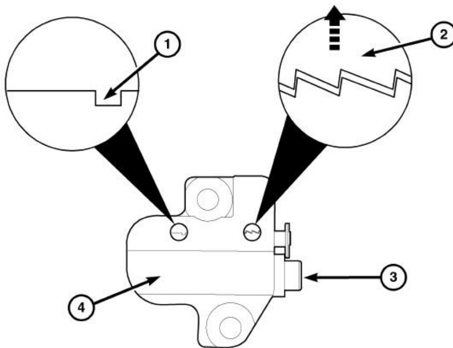
Fig. 400: Tensioner Reset
