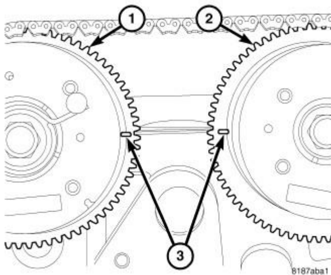
Fig. 365: Camshaft Timing Marks
