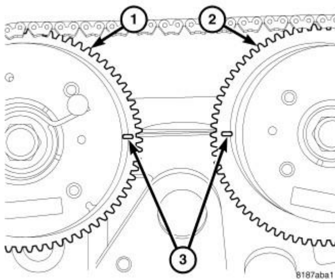
Fig. 350: Camshaft Timing Marks
