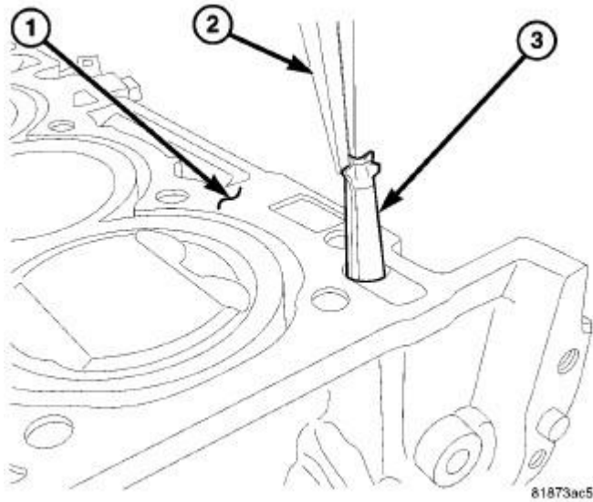
Fig. 269: VVT Filter
