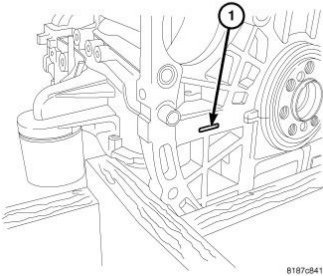
Fig. 216: Pry Point 1
