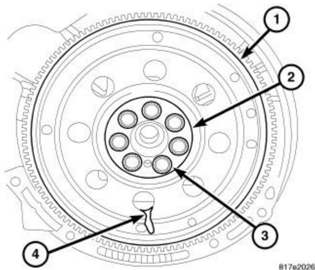
Fig. 214: Flex Plate
