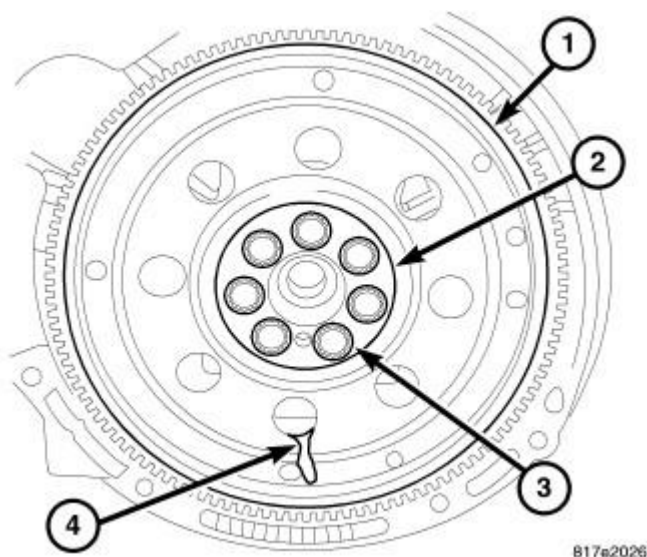
Fig. 215: Flex Plate
