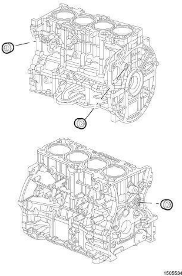
Fig. 299: Tapered Plugs
