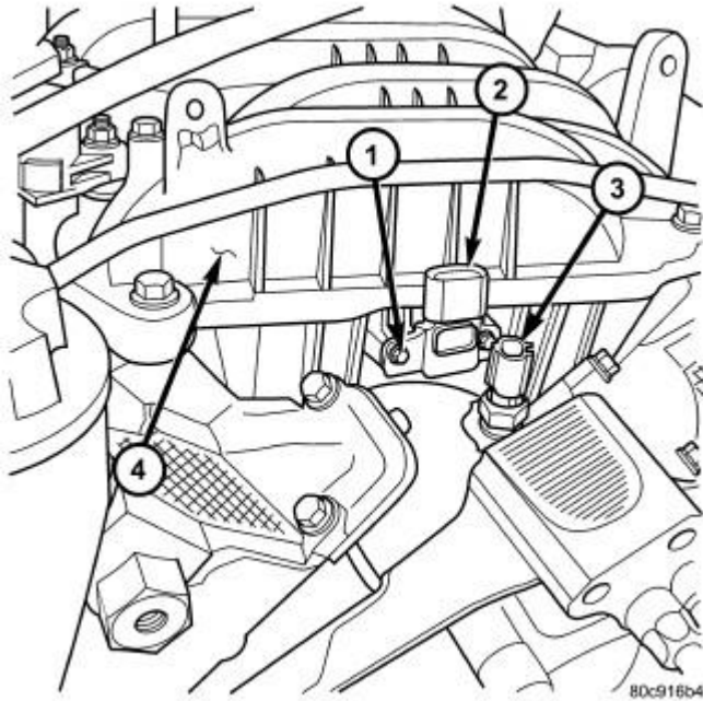
Fig. 167: MAP SENSOR - 3.7L V-6
