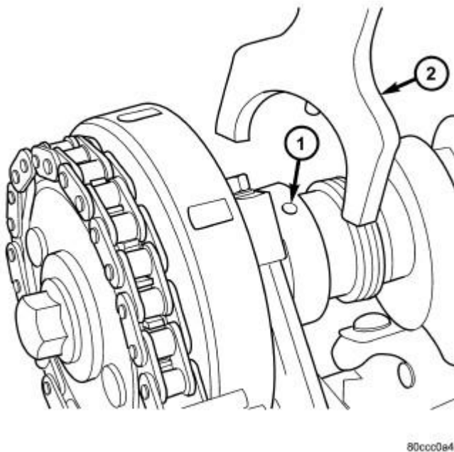
Fig. 56: Camshaft & Camshaft Holder
