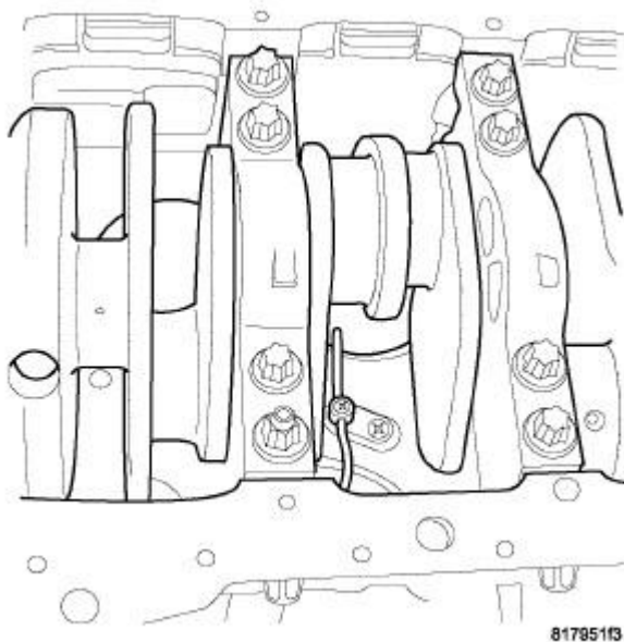
Fig. 335: OIL JET
