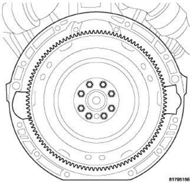
Fig. 362: FLEX PLATE
