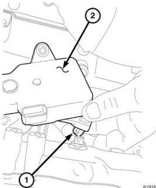
Fig. 477: INSTALL CLIP
