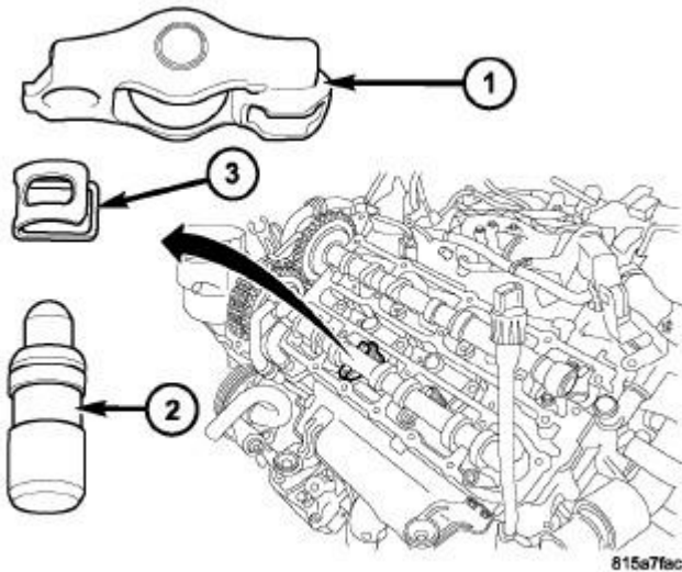
Fig. 277: ROCKER ARMS
