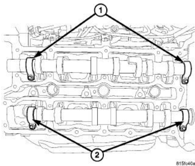
Fig. 162: CAMSHAFT RETAINERS
