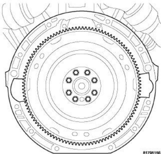
Fig. 361: Flex Plate
