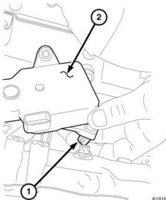
Fig. 477: INSTALL CLIP
