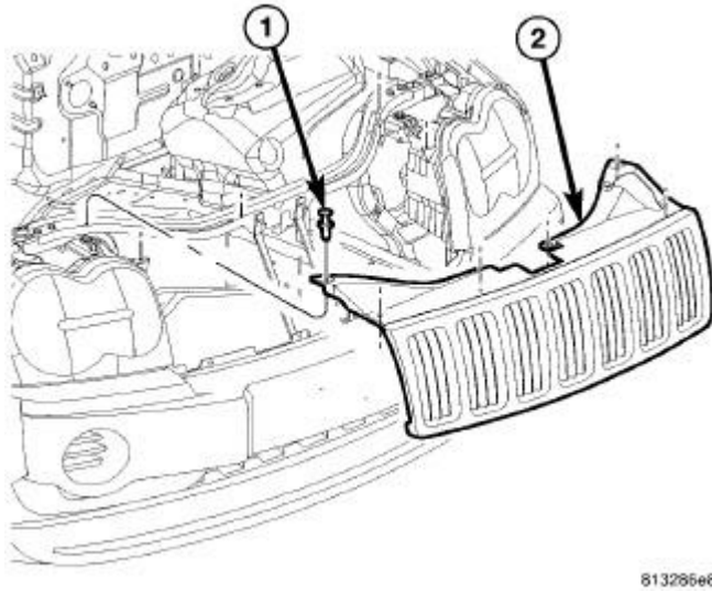
Fig. 9: GRILLE
