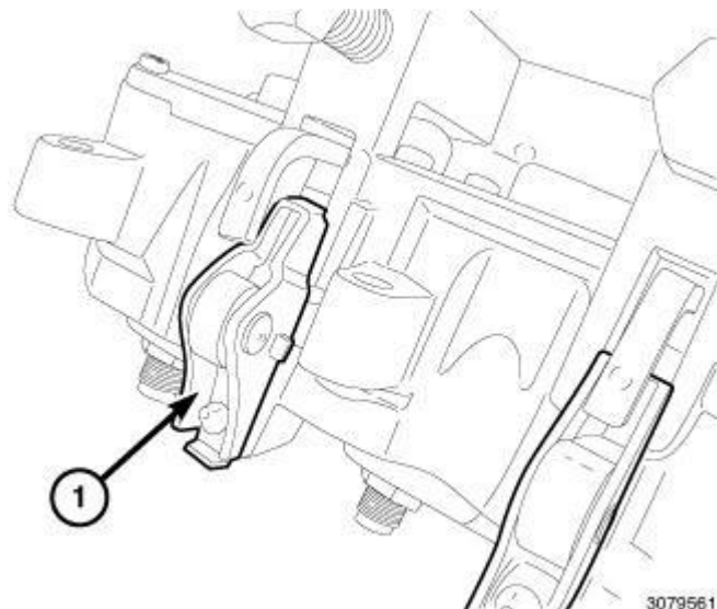
Fig. 189: Rocker Arms
