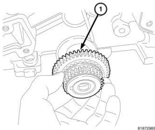
Fig. 407: Crankshaft Sprocket
