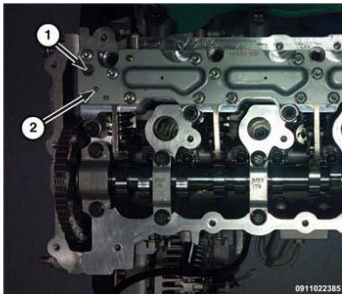
Fig. 199: Service Port & Bleed Port
