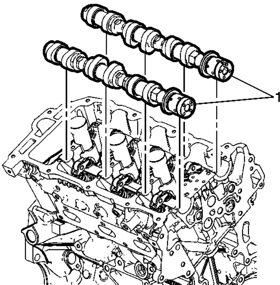
Fig. 154: Camshafts
