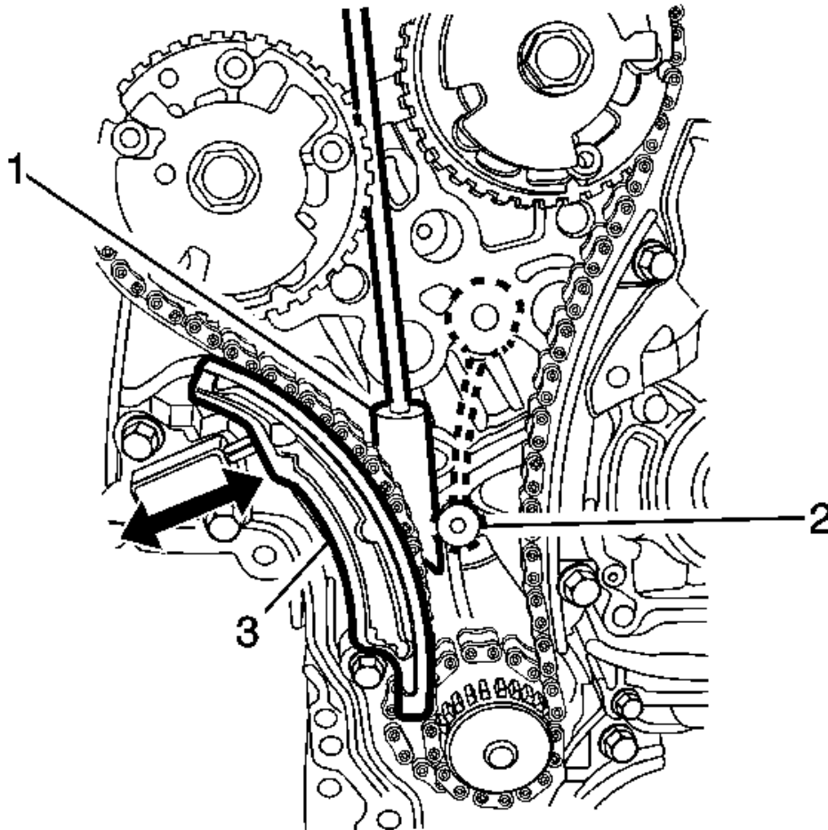
Fig. 110: Retainer Wedge
