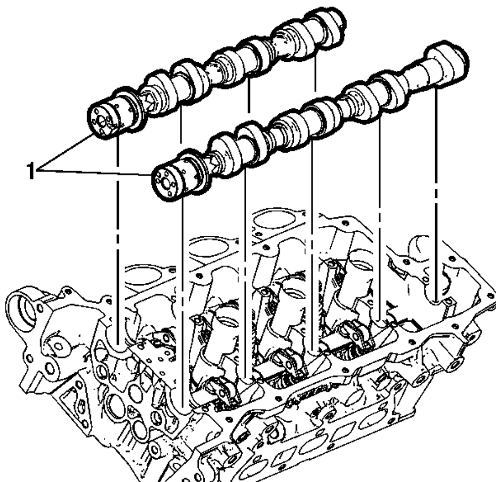
Fig. 157: Camshafts
