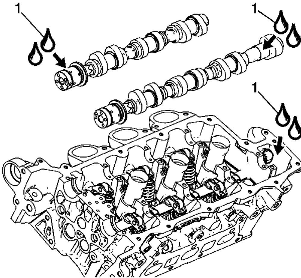
Fig. 159: Camshaft Journal Lubrication Points
