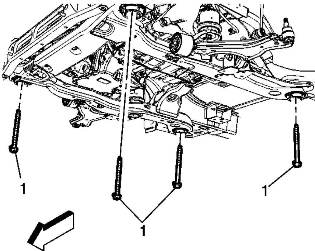
Fig. 265: Frame-To-Body Bolts
