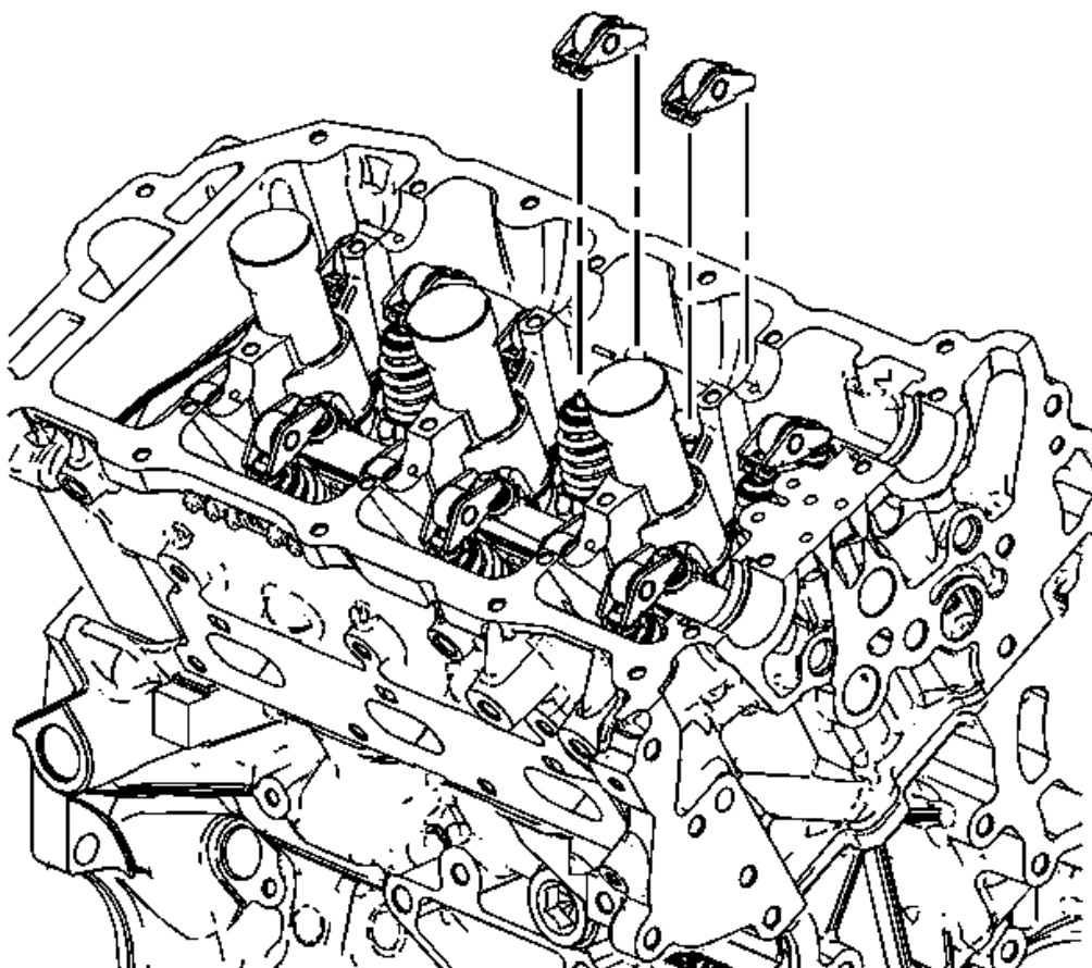
Fig. 177: Valve Rocker Arms
