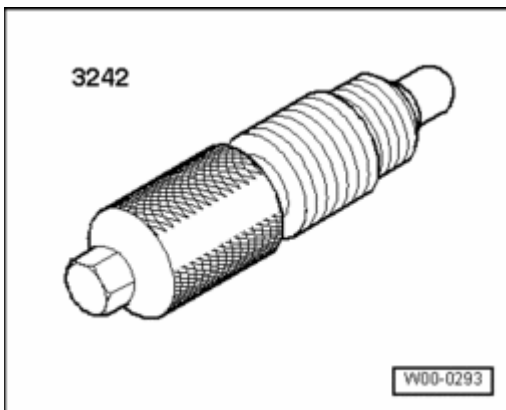
Fig. 342: Locking Pin 3242
