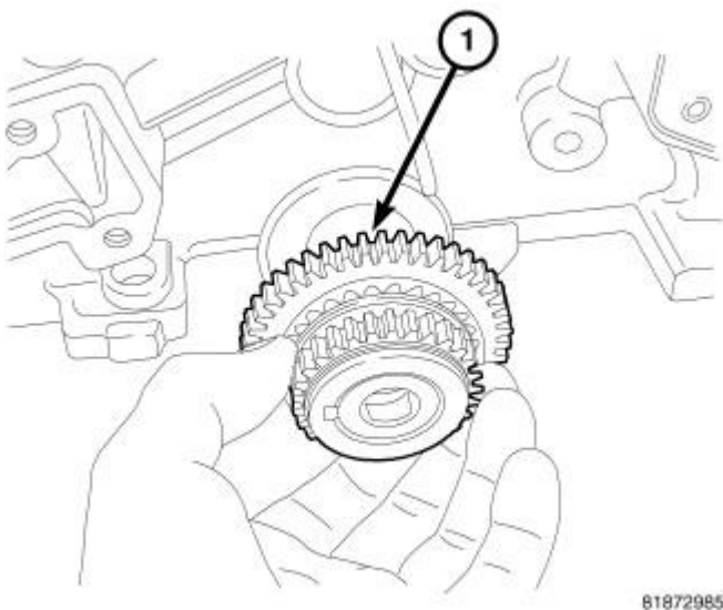
Fig. 329: CRANKSHAFT SPROCKET
