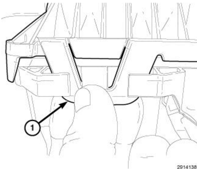
Fig. 57: Air Box Lid Tabs
