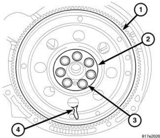
Fig. 203: FLEX PLATE
