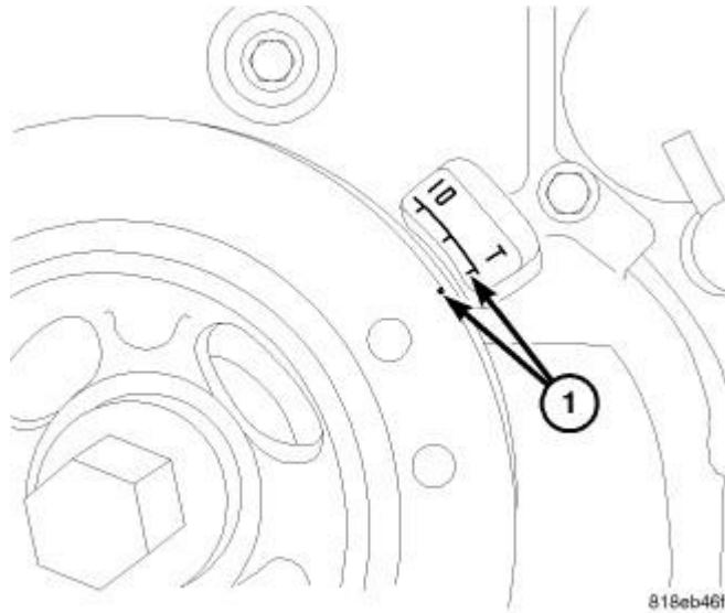
Fig. 68: TDC
