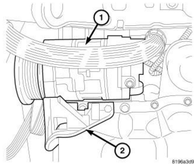
Fig. 69: A/C COMPRESSOR
