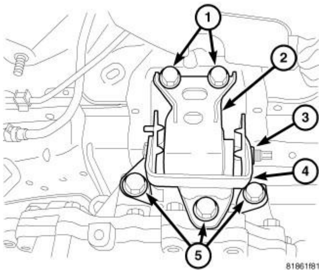
Fig. 233: LEFT MOUNT
