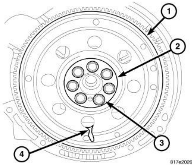
Fig. 179: FLEX PLATE
