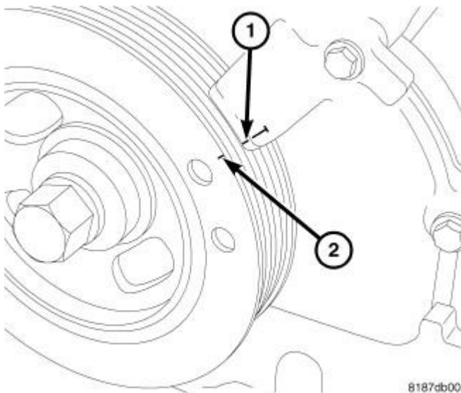
Fig. 322: TDC
