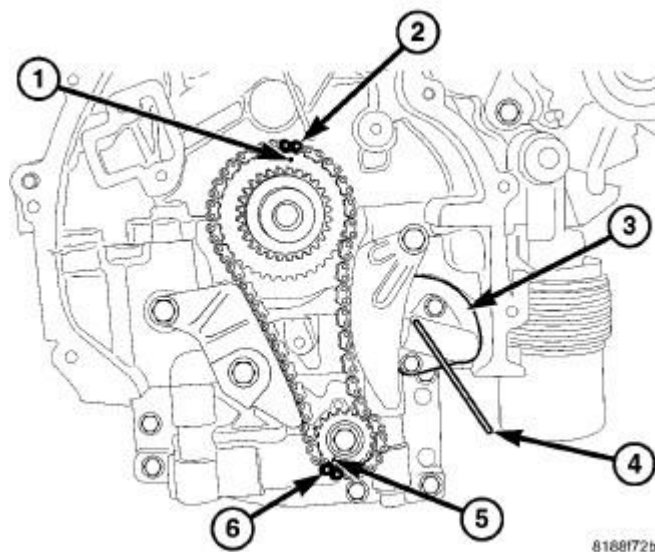
Fig. 287: BSM TENSIONER
