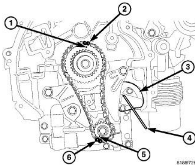
Fig. 285: BSM TENSIONER
