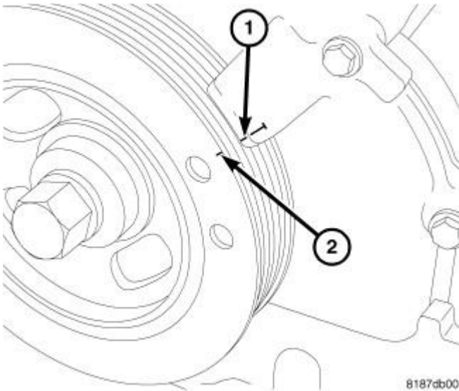
Fig. 284: TDC
