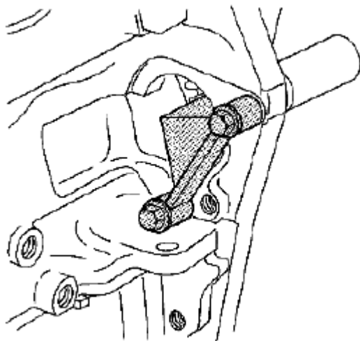
Fig. 96: Identifying Special Tool (EN 46106) Courtesy of SUZUKI OF AMERICA CORP.
