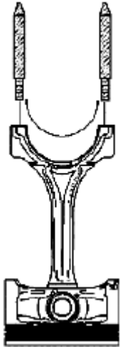
Fig. 380: Identifying Special Tool (EN 46121) Courtesy of SUZUKI OF AMERICA CORP.
