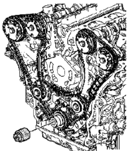
Fig. 307: Identifying Special Tool (EN 46111) Courtesy of SUZUKI OF AMERICA CORP.
