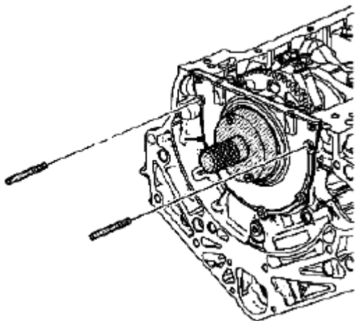
Fig. 738: Identifying Special Tool (EN 46109) Courtesy of SUZUKI OF AMERICA CORP.
