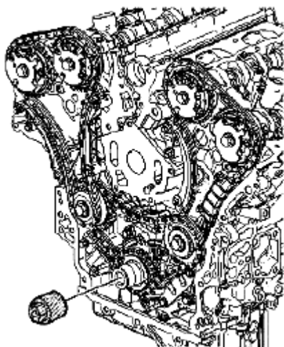
Fig. 297: Identifying Special Tool (EN 46111) Courtesy of SUZUKI OF AMERICA CORP.
