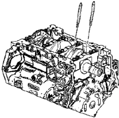
Fig. 727: Identifying Special Tool (EN 46121) Courtesy of SUZUKI OF AMERICA CORP.
