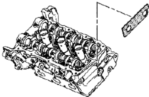
Fig. 893: Identifying Special Tool (EN 46105-1) Courtesy of SUZUKI OF AMERICA CORP.
