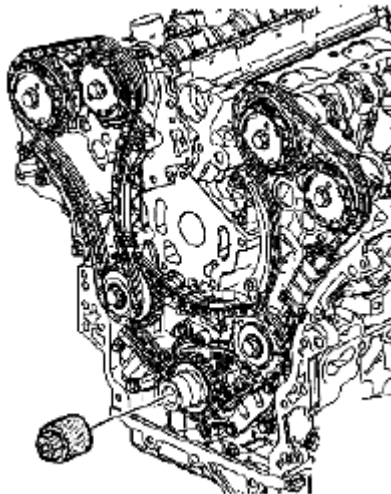
Fig. 118: Identifying Special Tool (EN 46111) Courtesy of SUZUKI OF AMERICA CORP.
