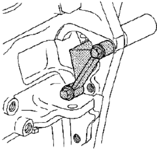
Fig. 195: Identifying Special Tool (EN 46106) Courtesy of SUZUKI OF AMERICA CORP.
