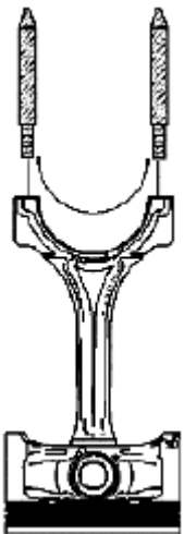
Fig. 437: Identifying Special Tool (EN 46121) Courtesy of SUZUKI OF AMERICA CORP.
