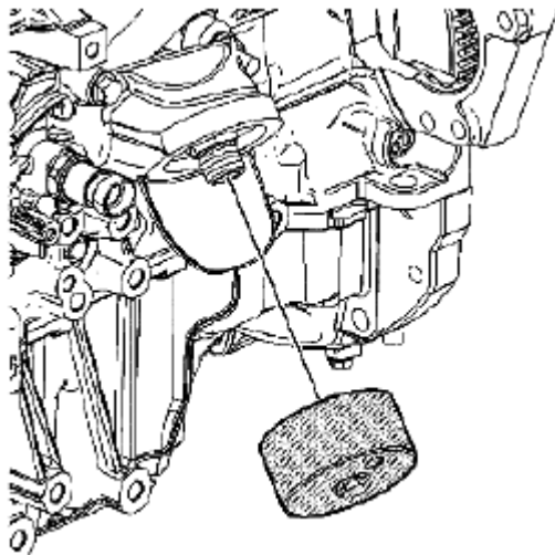
Fig. 1004: Identifying Special Tool (EN 47971) Courtesy of SUZUKI OF AMERICA CORP.
