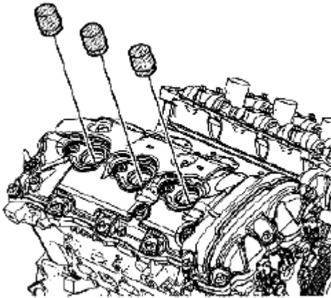
Fig. 977: Identifying Special Tool (EN 46101) Courtesy of SUZUKI OF AMERICA CORP.
