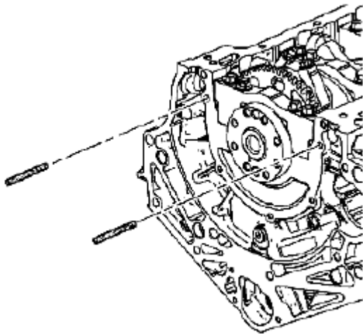
Fig. 734: Identifying Special Tool (EN 46109) Courtesy of SUZUKI OF AMERICA CORP.
