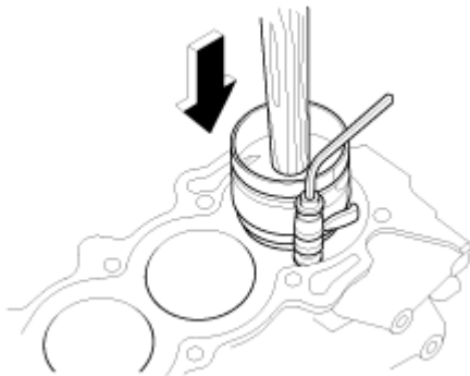
Fig. 37: Installing Piston
