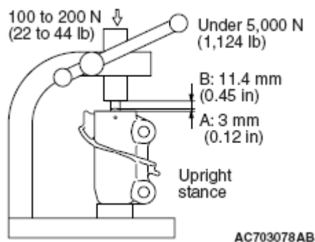
Fig. 100: Checking Auto-Tensioner
