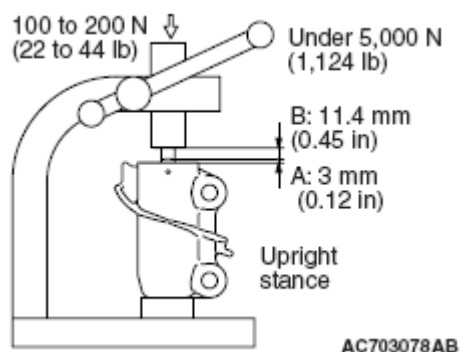
Fig. 97: Setting Auto-Tensioner
