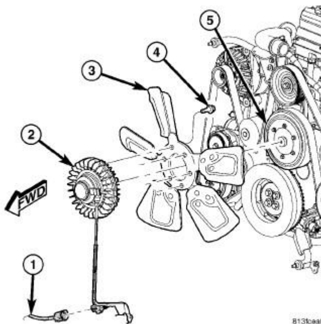
Fig. 355: Fan Blade/Viscous Fan Drive - 5.9L Diesel Courtesy of CHRYSLER LLC
