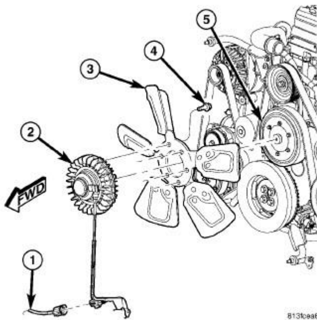
Fig. 350: Fan Blade/Viscous Fan Drive Courtesy of CHRYSLER LLC
