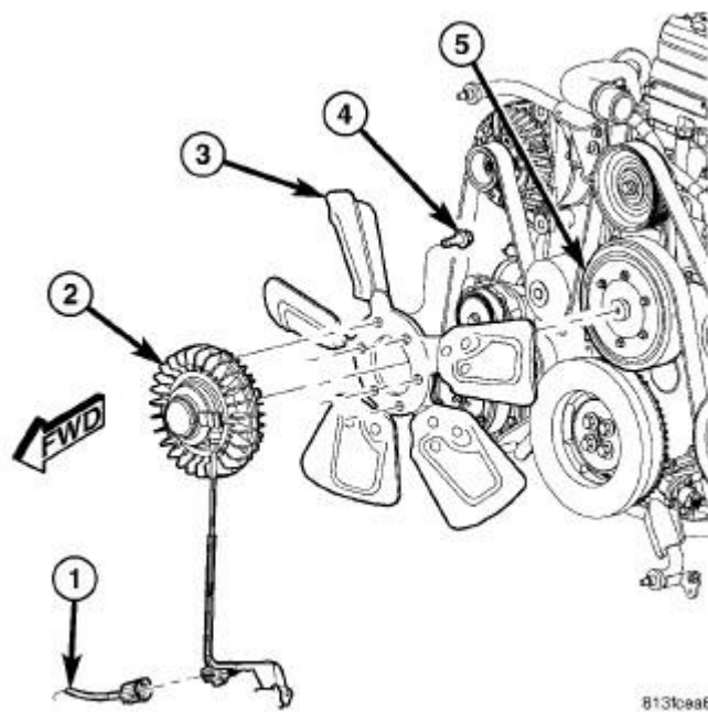
Fig. 353: Fan Blade/Viscous Fan Drive - 5.9L Diesel Courtesy of CHRYSLER LLC
