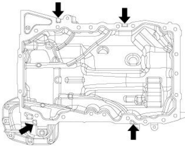
Fig. 576: Pry Points
