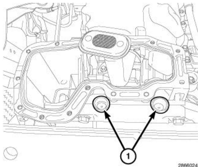
Fig. 586: Rubber Plugs
