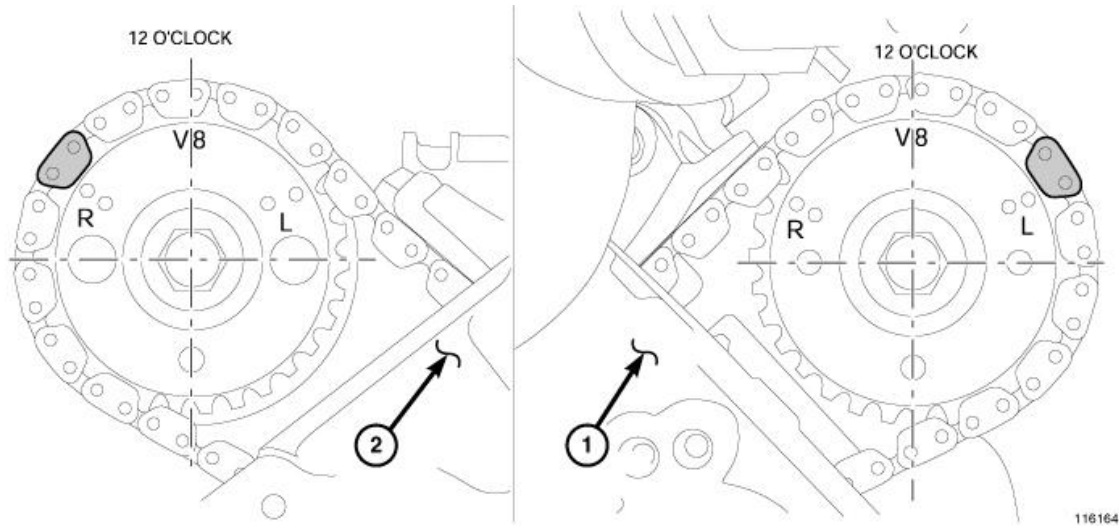
Fig. 215: Camshaft Sprocket V8 Marks Courtesy of CHRYSLER LLC
