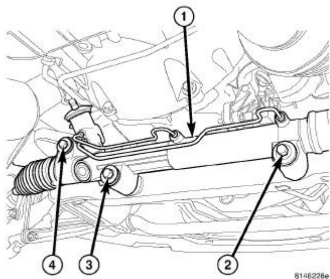
Fig. 338: AWD Gear Mounting Bolts
