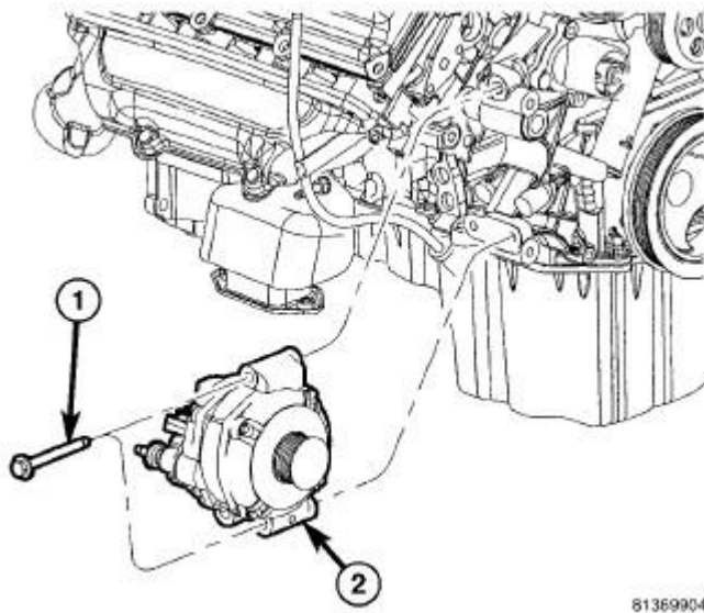
Fig. 24: Generator - 5.7L
