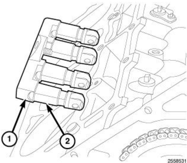
Fig. 215: Tappet Guide Holder Assembly
