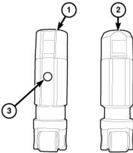
Fig. 76: MDS Lifter
