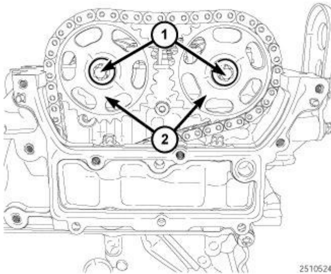
Fig. 642: Camshaft Sprockets & Bolts Courtesy of CHRYSLER LLC
