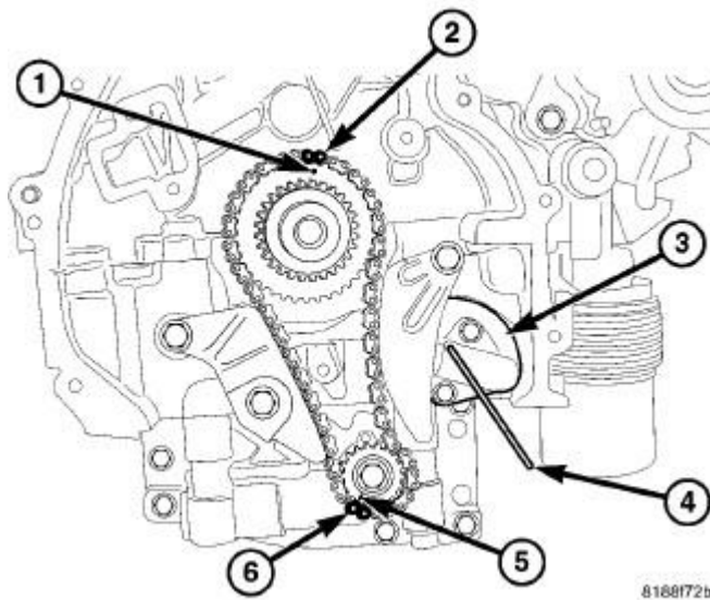
Fig. 295: BSM Tensioner
